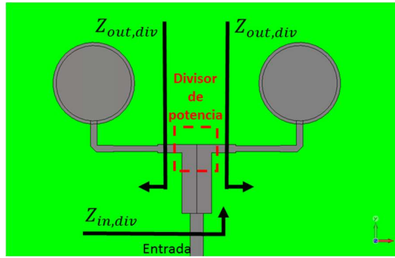
Figura 3.6. Vista superior de un divisor de potencia microstrip con parches conectados a sus salidas.
