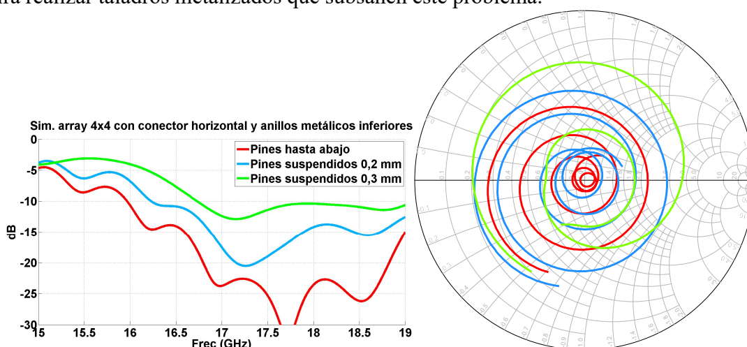
Figura 4.11. Evolución de la adaptación conforme el pin de acoplo de la SIW a la microstrip no llega a quedar a ras del plano de masa inferior de la SIW.
