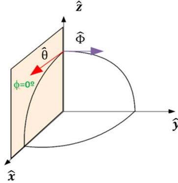
Figura 2.5. Vectores unitarios \hat{\theta} y \hat{\phi} para \phi = 0^\circ
