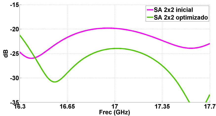
Figura 3.10. Coeficiente de adaptación del subarray 2x2 antes y después de optimizar la estructura completa.
