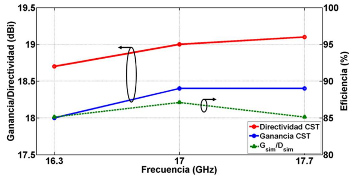
Figura 3.21. Evaluación de directividad y ganancia simuladas en el array 4x4.
