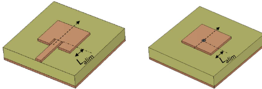
Figura 2.11. Parche rectangular alimentado mediante línea microstrip (izquierda) y parche rectangular alimentado por sonda coaxial vertical (derecha). Imagen extraída de [15].
