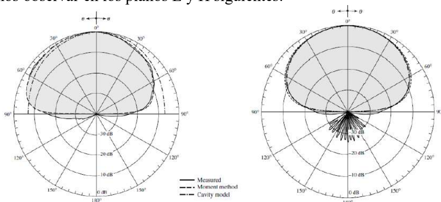
Figura 2.15. Diagrama de radiación del parche circular en el plano E ( \phi = 0^\circ , izd) y el plano H ( \phi = 90^\circ , dcha).
